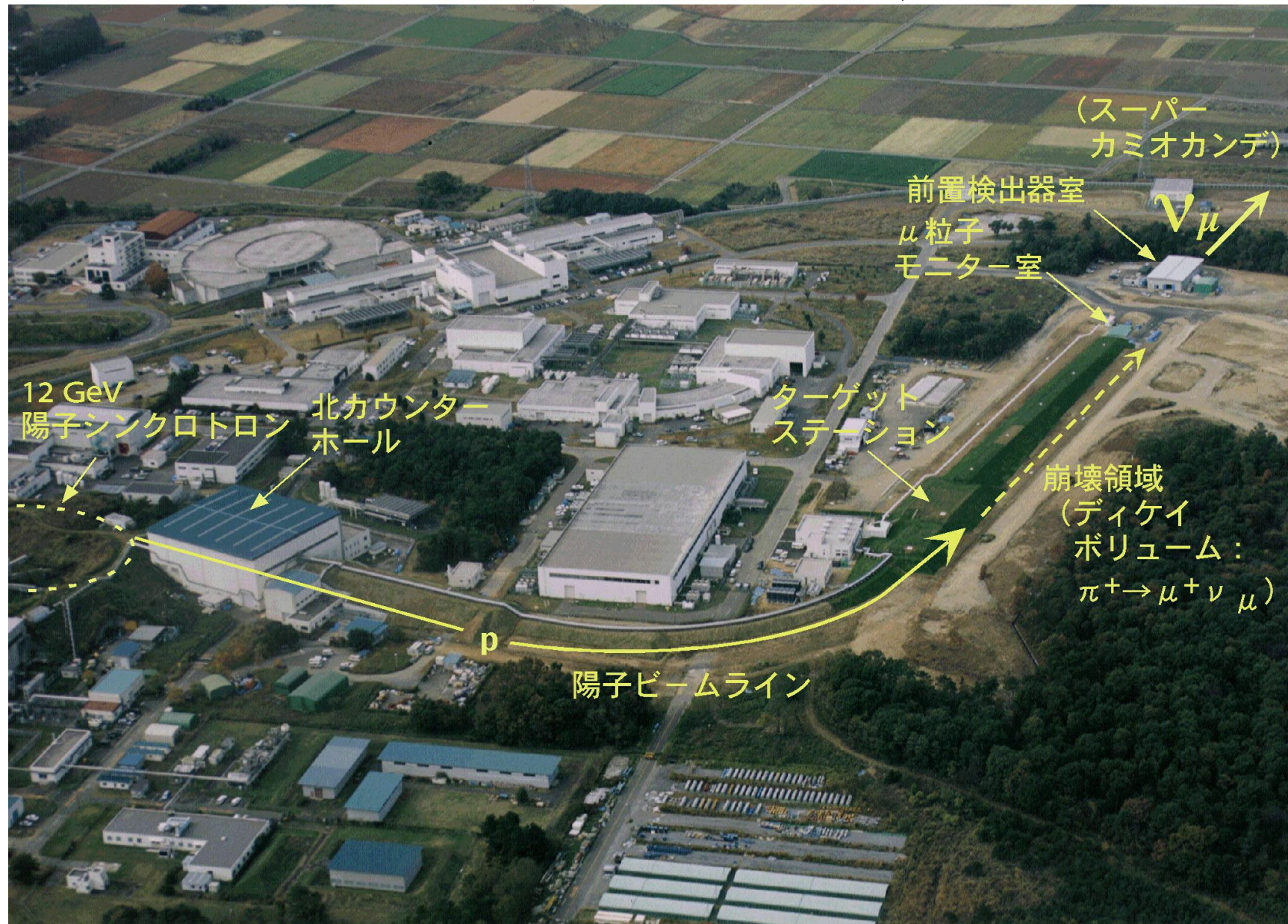
ニュートリノビームライン全景
