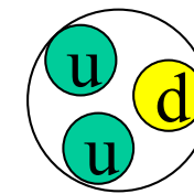
陽子
