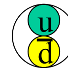
π中間子
