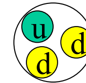
中性子
